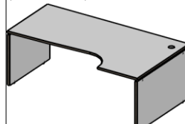
ДБ08 Стол Правый (1600x900x750)
